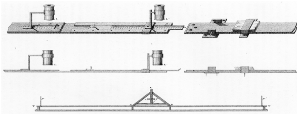
APPAREIL DES BASES DE BORDA... d'après PUISSANT
